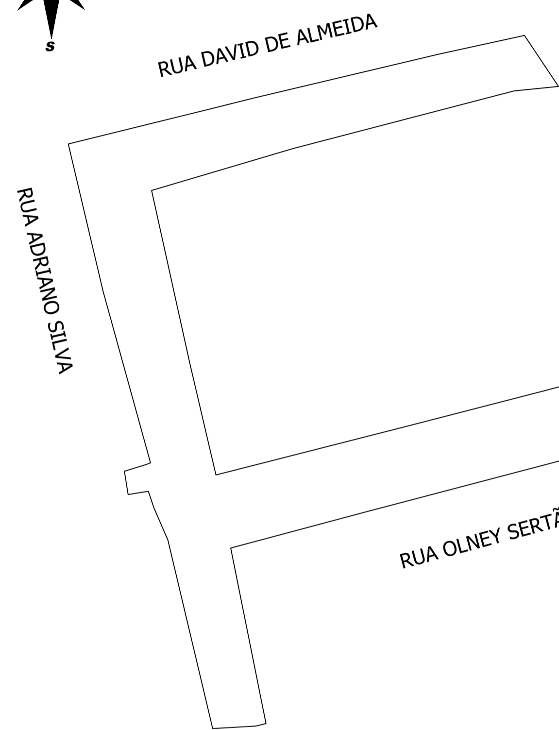
LOCAÇÃO DRENAGEM PLUVIAL ESCALA:.....1 / 500
