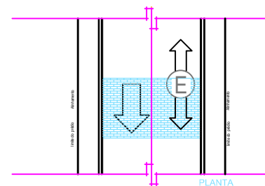
DETALHE 2 DISTRIBUIÇÃO DE FLUXO DE VEÍCULOS ESC.: S/ESC COT.: METROS
