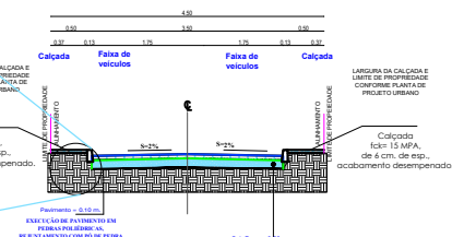
DETALHE CONSTRUTIVO TIPO SEÇÃO 2 PISTAS
