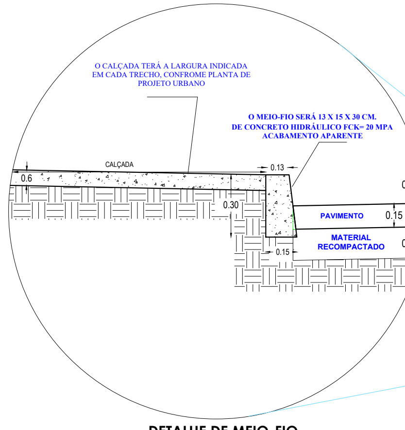
DETALHE DE MEIO-FIO E CALÇADA ESC. 5/ESC. COT.: METROS
