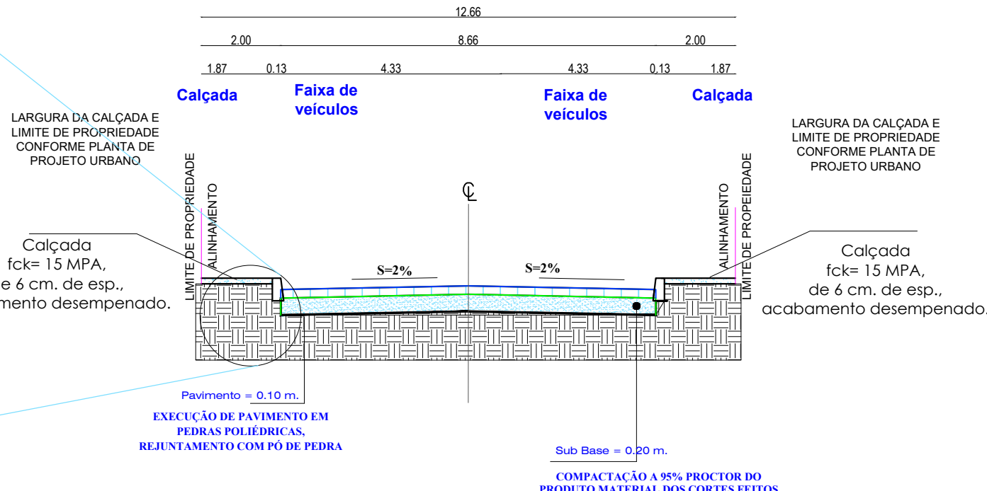
DETALHE CONSTRUTIVO TIPO SEÇÃO 2 PISTAS ESC. 5/ESC. COT.: METROS
