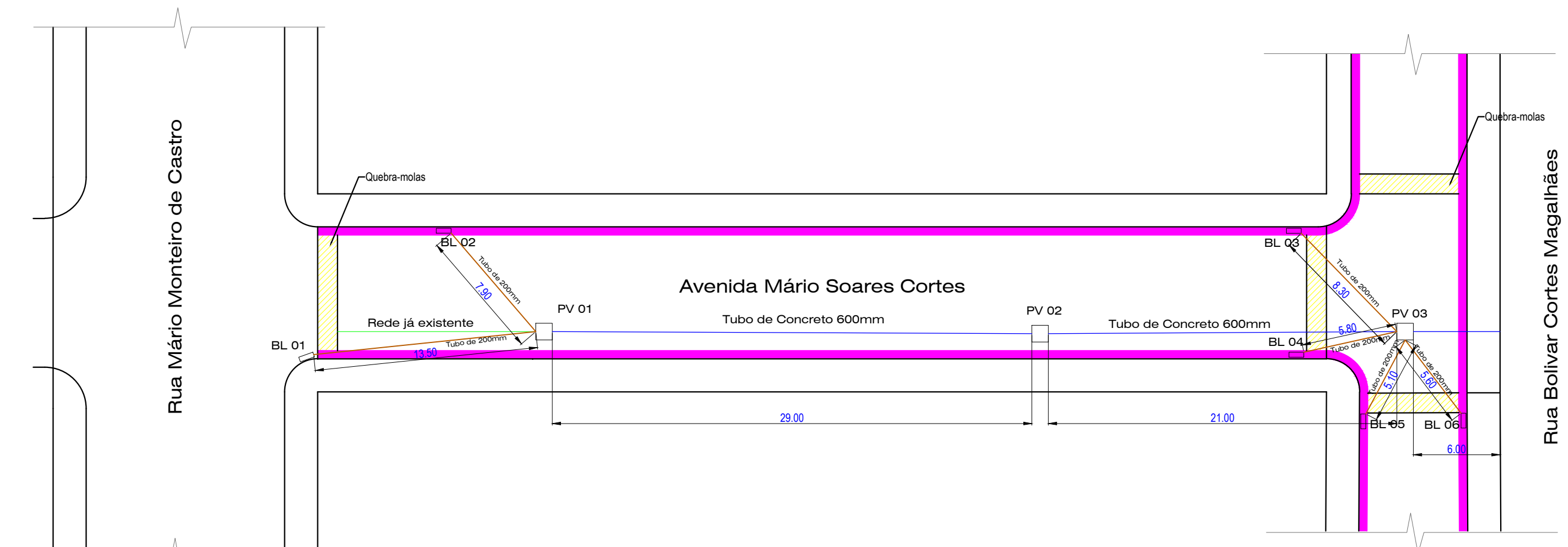
PLANTA DE SITUAÇÃO - DRENAGEM PLUVIAL ESCALA 1/250
