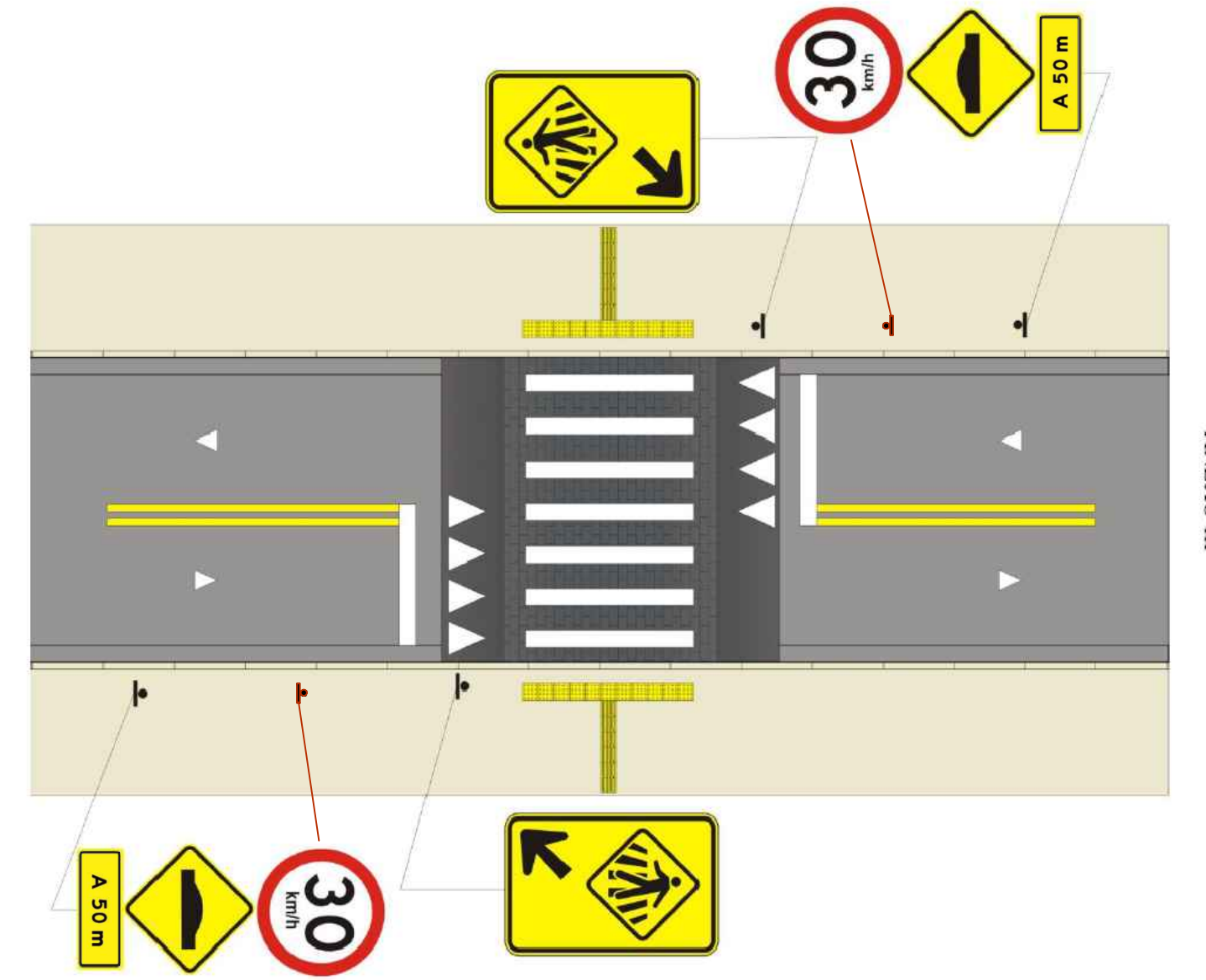
PLACAS - FAIXA ELEVADA SEM ESCALA
