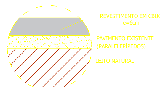
DETALHE 2 SEM ESCALA
