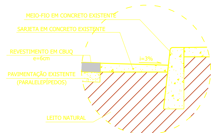
DETALHE 1 SEM ESCALA
