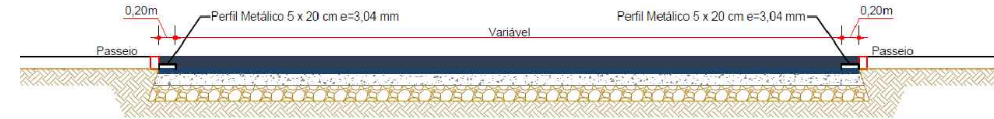
CORTE BB - FAIXA ELEVADA SEM ESCALA
