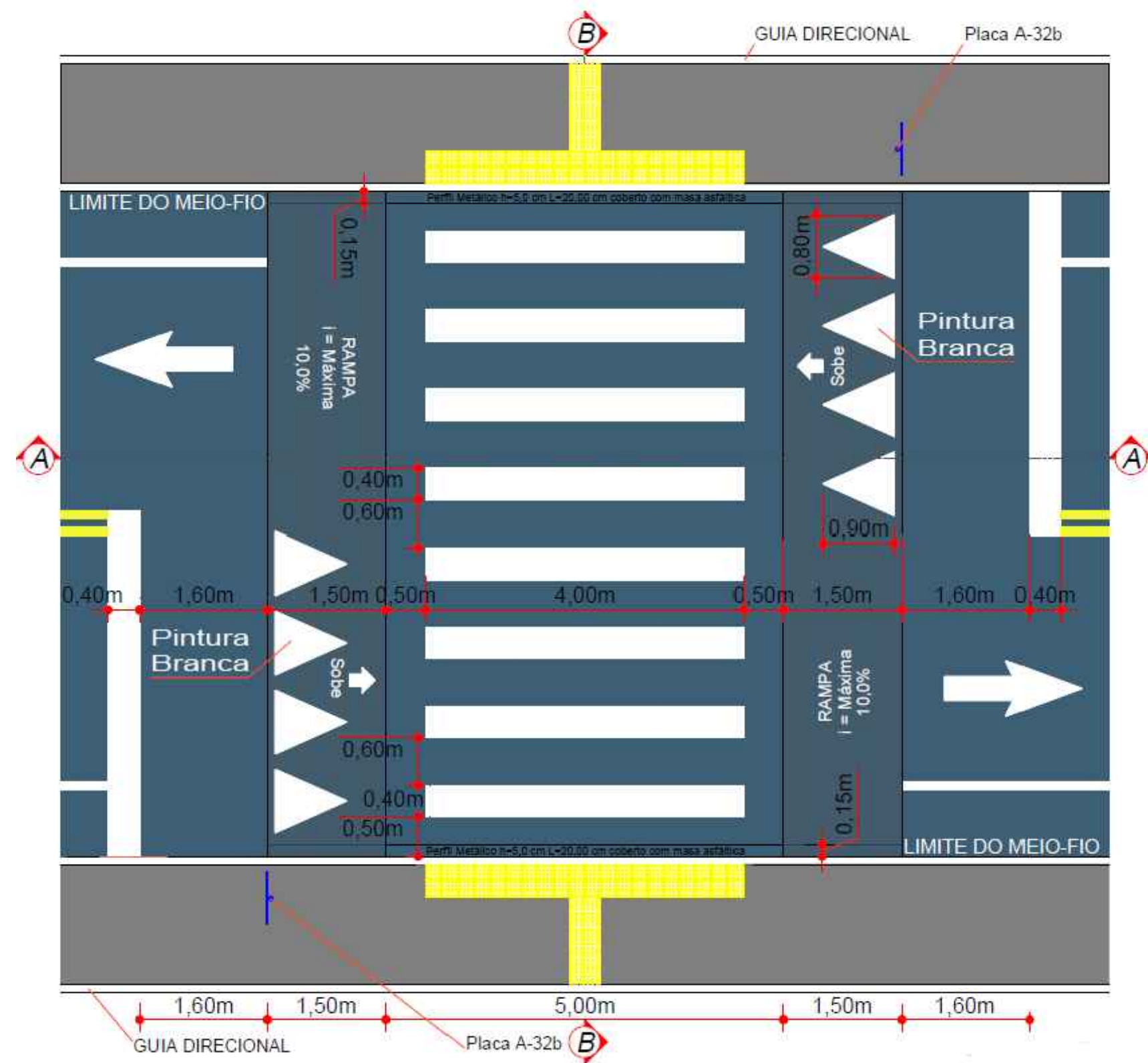
PLANTA BAIXA - FAIXA ELEVADA (VIDE NOTA Nº 4) SEM ESCALA
