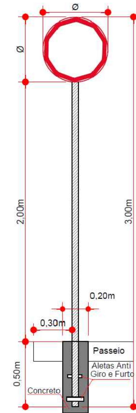
FIXAÇÃO DAS PLACAS SEM ESCALA
