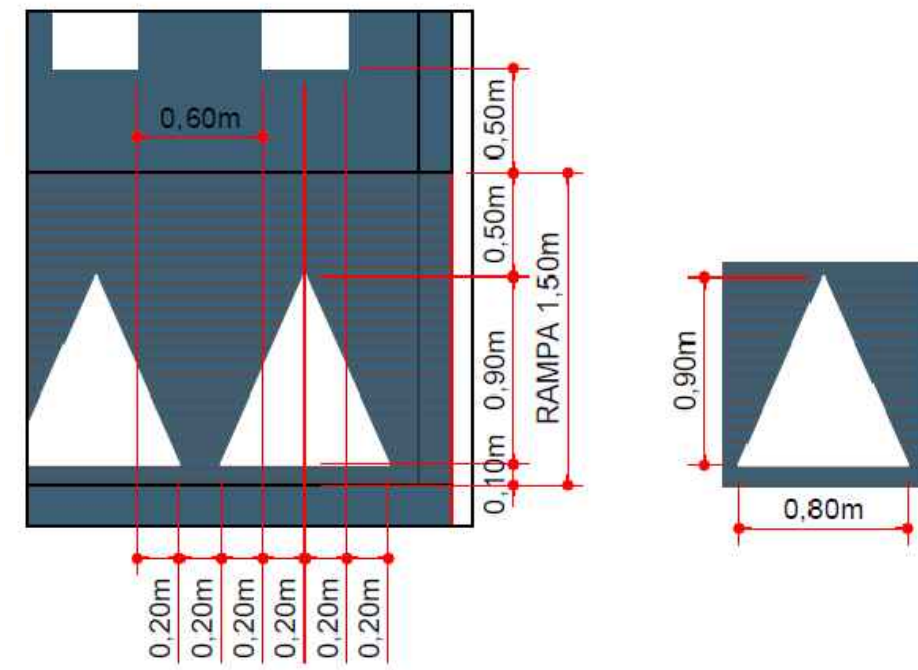
SINALIZAÇÃO HORIZONTAL SEM ESCALA
