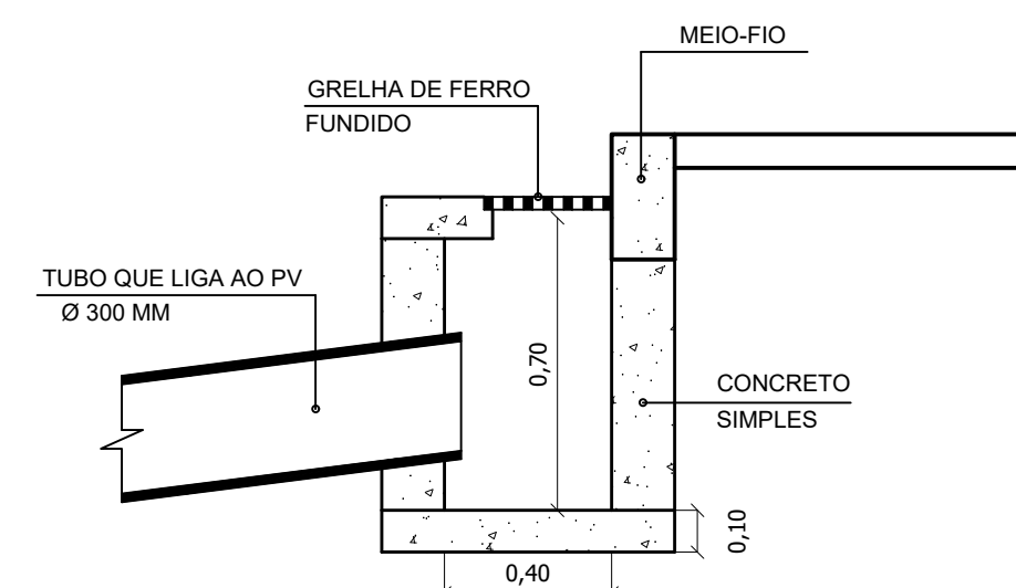
CORTE A-A - BL ESCALA:.....1 / 20
