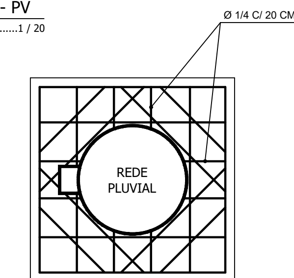
TAMPA - ARMAÇÃO - PV ESCALA:.....1 / 20
