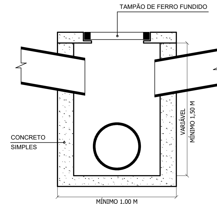
CORTE A-A - PV ESCALA:.....1 / 20
