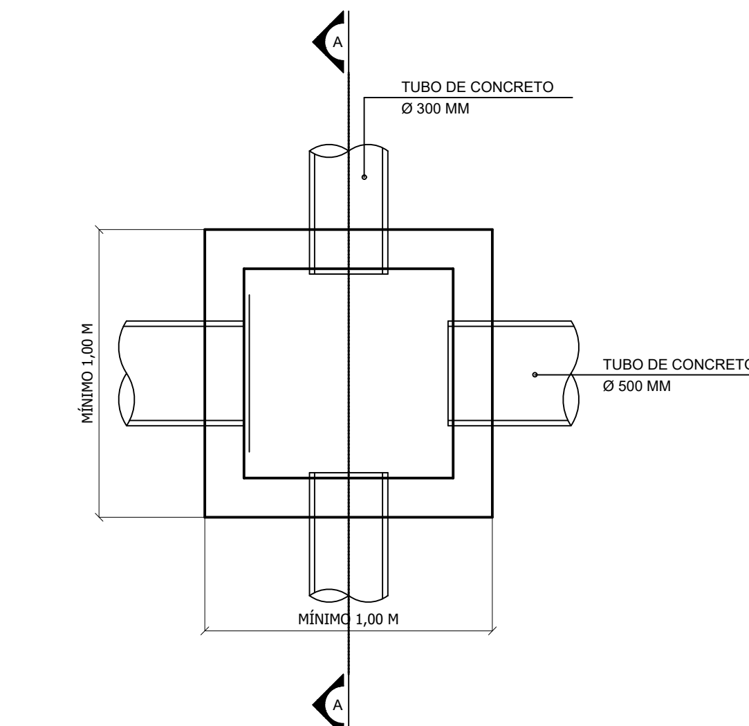
PLANTA BAIXA - PV ESCALA:.....1 / 20
